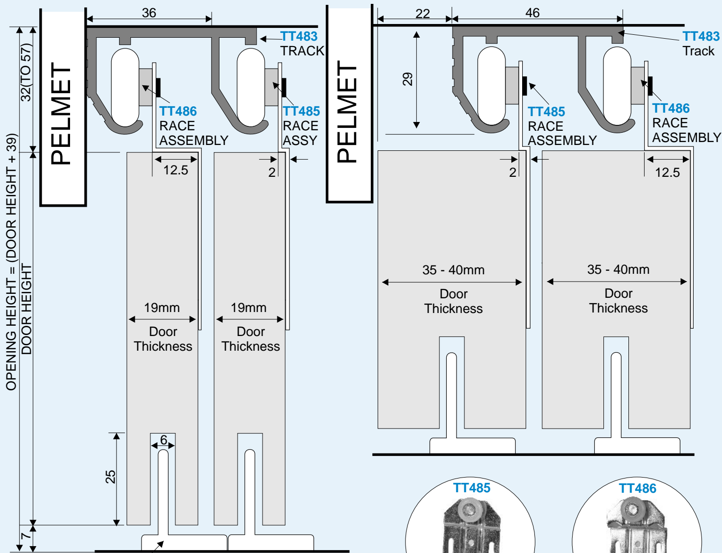
TT208 DOOR GUIDE
